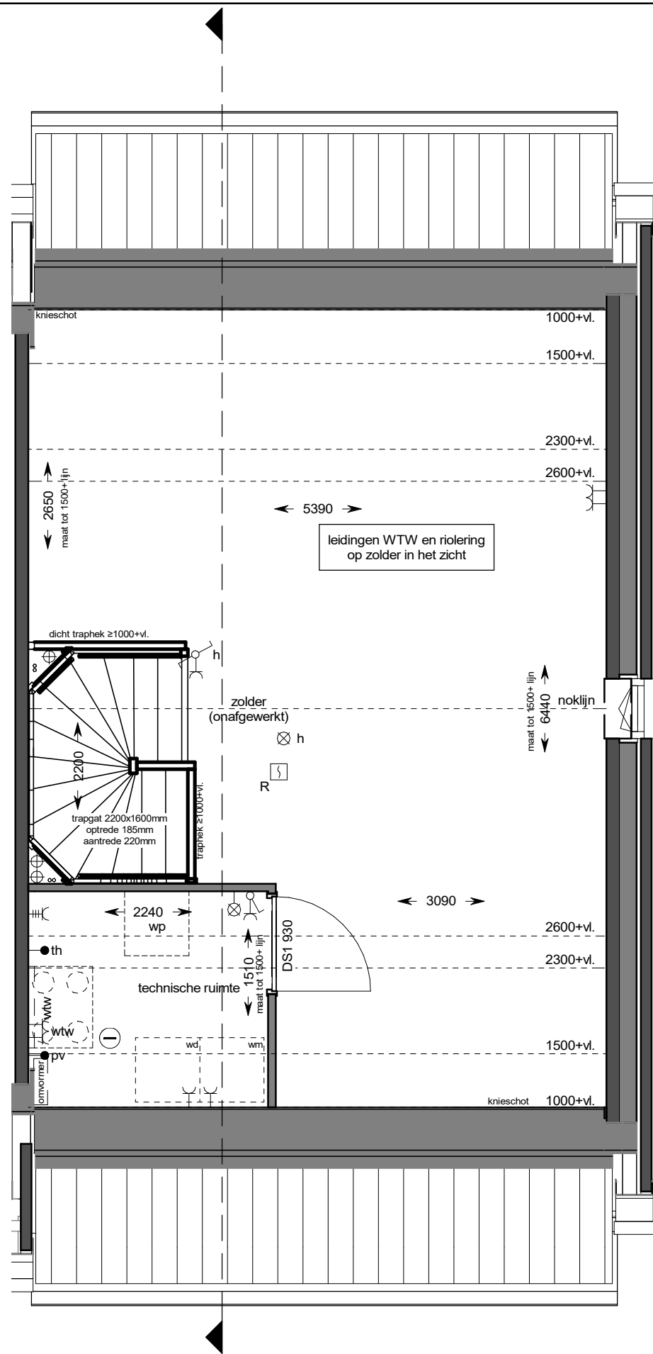
tweede verdieping
