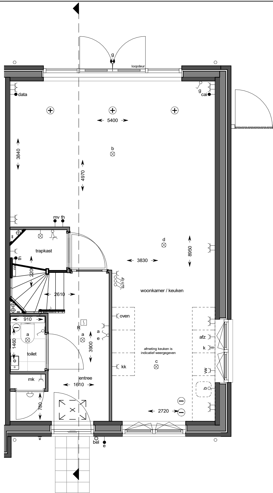
begane grond
