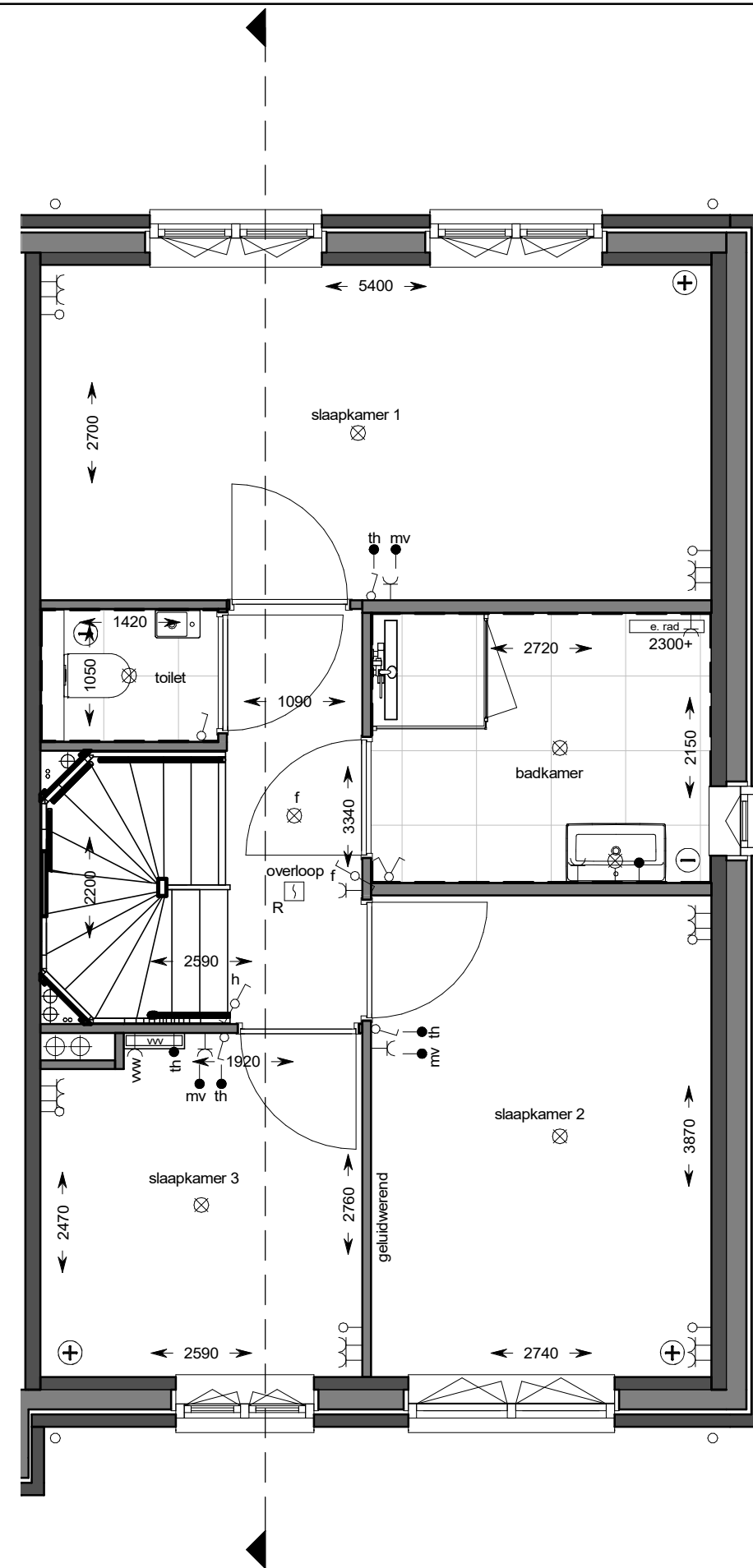
eerste verdieping
